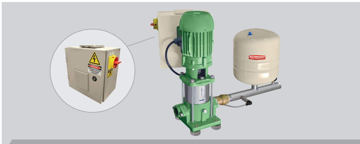
Sistema de pressurização acionado por inversor de frequência.
